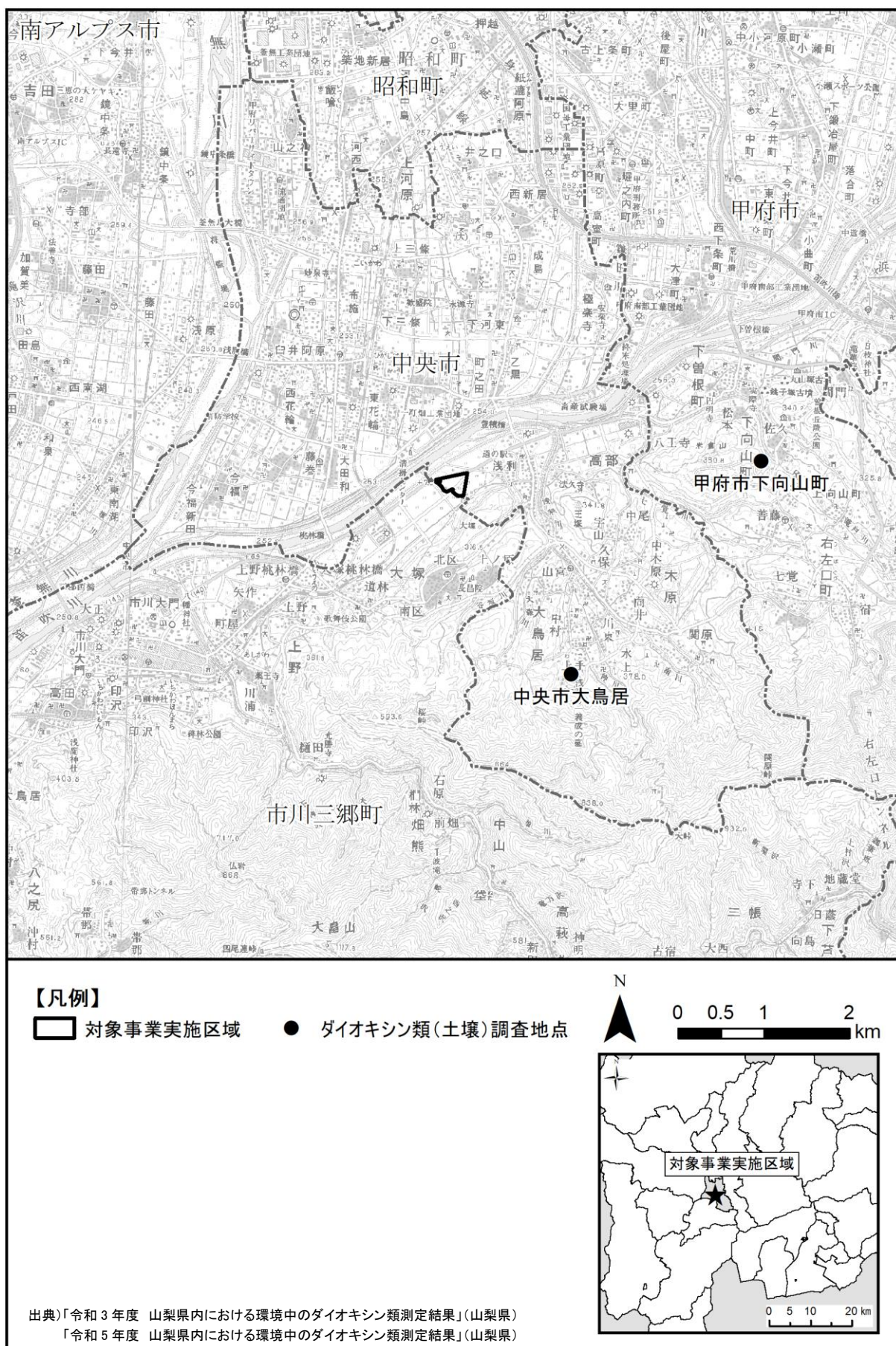
図 4.3-34 土壌（ダイオキシン類）調査地点
