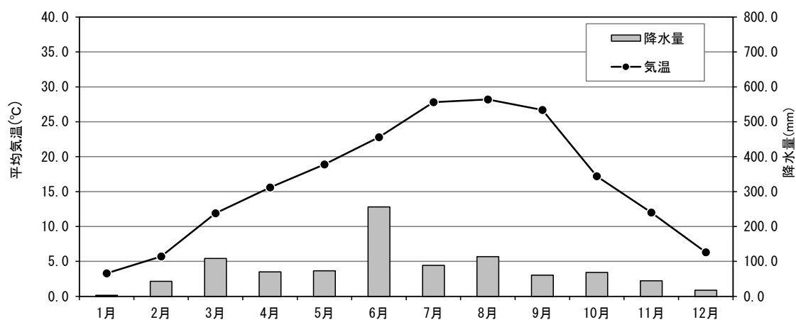
図4.2-2 甲府地方気象台の気温・降水量の推移(令和5年)
