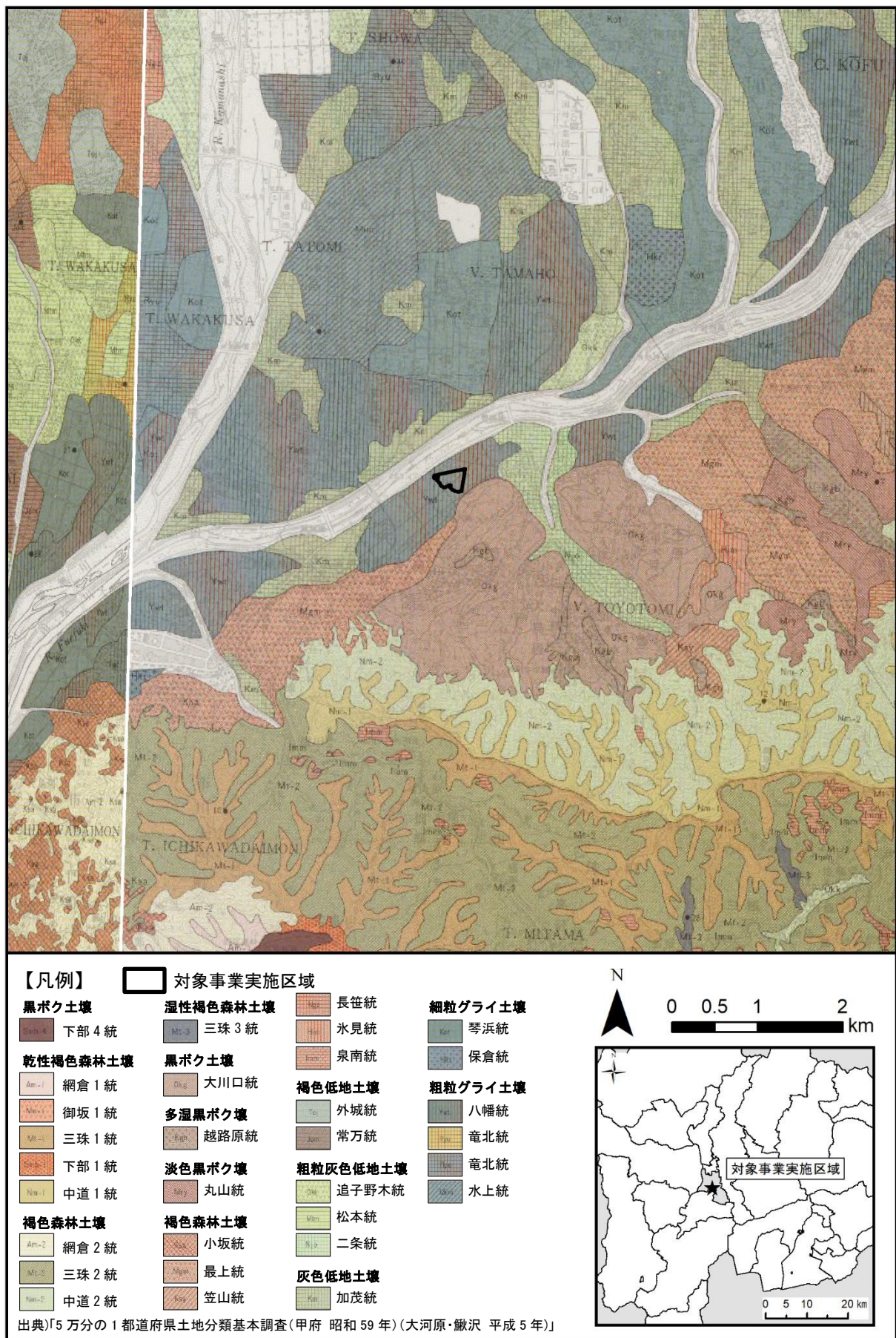
図 4.2-13 土壌図
