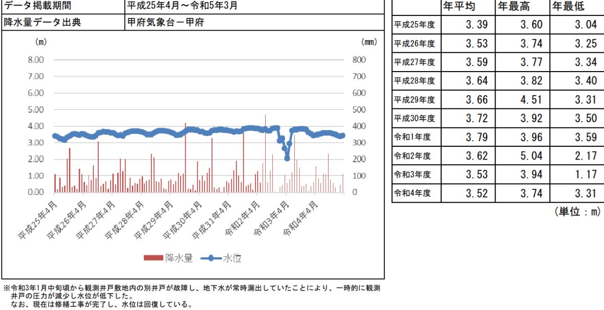
図 4.3-33 地下水位観測結果
