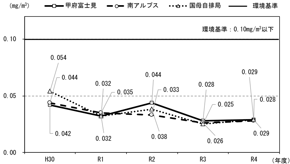
図 4.3-23 浮遊粒子状物質濃度の推移（年間2%除外値）
