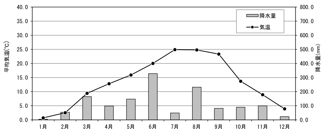
図4.2-5 古閑地域気象観測所の気温・降水量の推移(令和5年)
