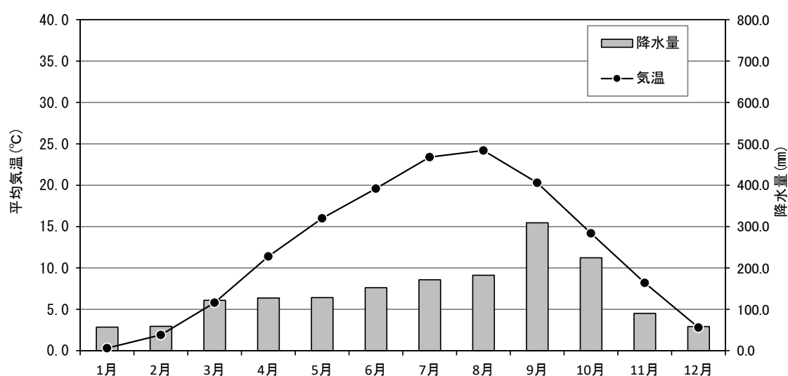
図 4.2-7 古関地域気象観測所の気温・降水量の推移（平年値）
