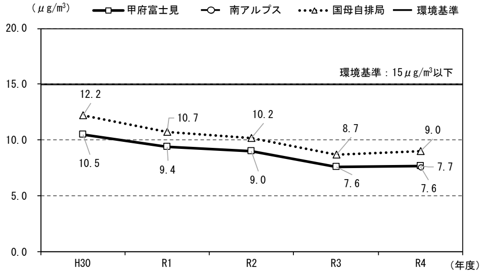
図 4.3-24(1) 微小粒子状物質濃度の推移 (1年平均値)
