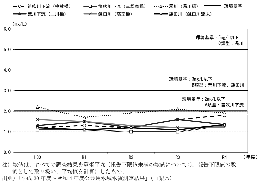
図 4.3-31 BOD の経年変化
