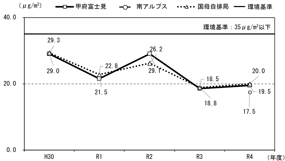
図 4.3-24(2) 微小粒子状物質濃度の推移 (1日平均値の年間98%値)
