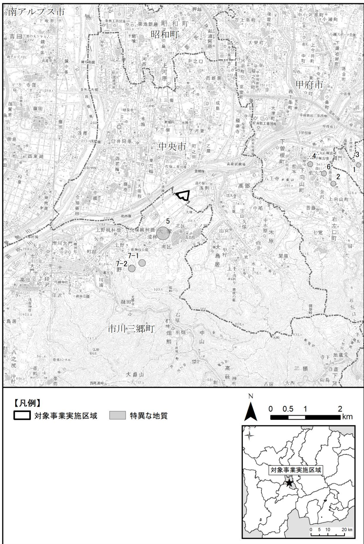
図 4. 2-12 特異な地質の分布
