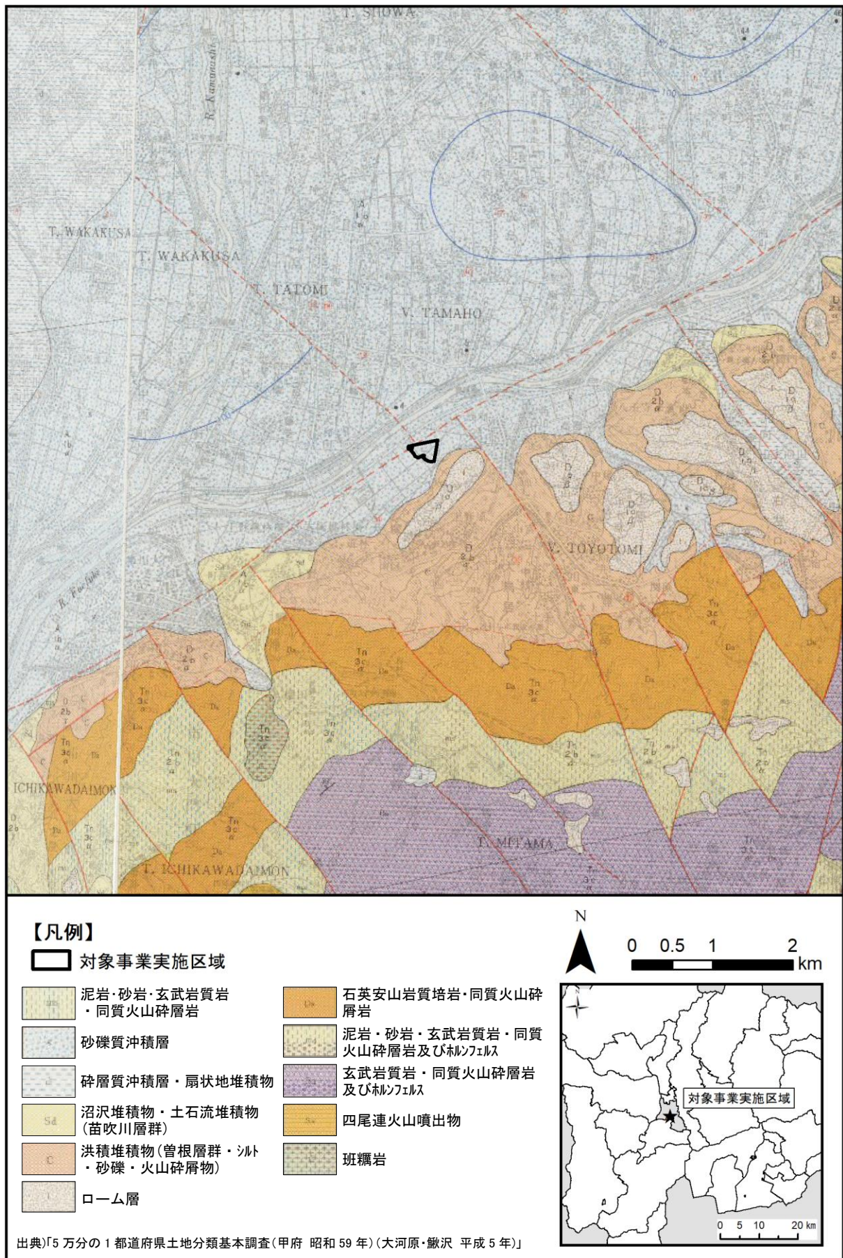
図 4.2-11 表層地質図
