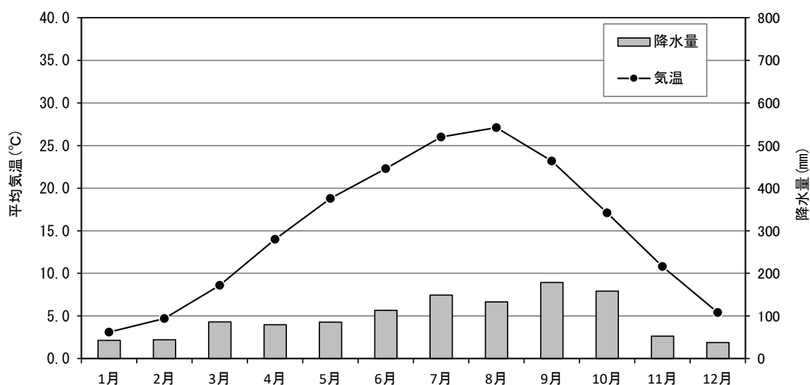
図 4.2-4 甲府地方気象台の気温・降水量の推移（平年値）
