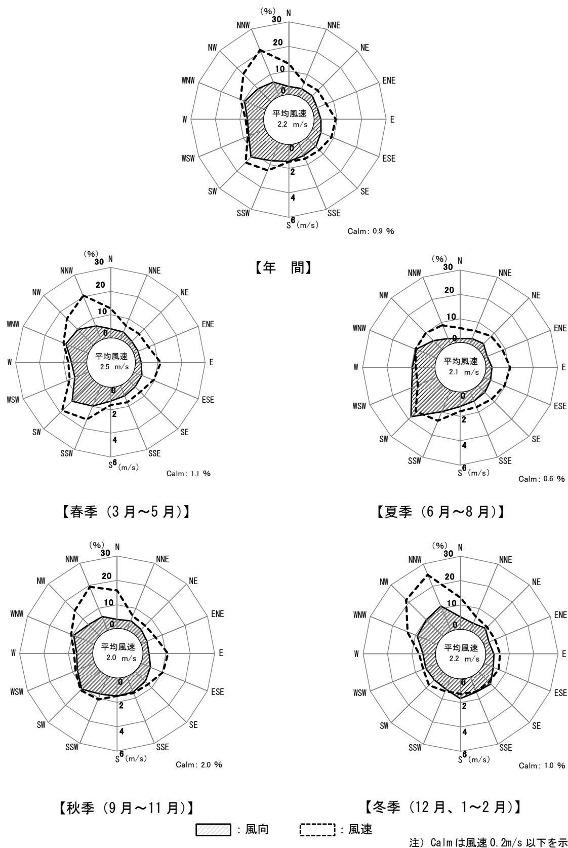
図 4.2-3 風向別出現頻度及び風向別平均風速（甲府地方気象台：令和 5 年）
