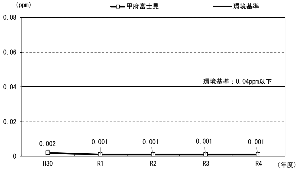
図 4.3-18 二酸化硫黄濃度の推移（年間 2%除外値）
